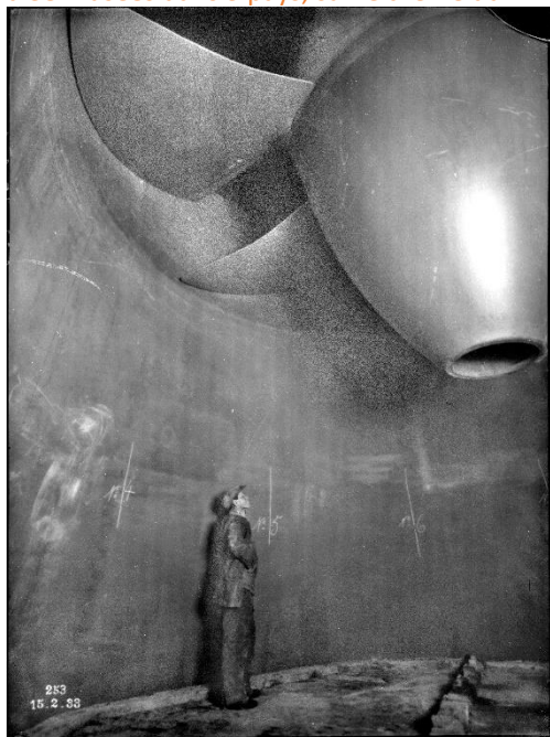
Hélice de l'une des cinq turbines, 1933.
